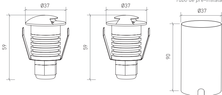
Pre-installation tube Tubo de pré-instalação
