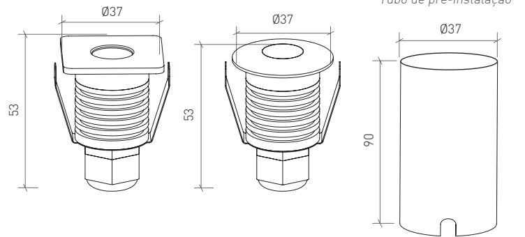
Pre-installation tube Tubo de pré-instalação
