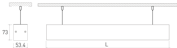
Suspension kit 1500mm . Kit de suspensão 1500mm
