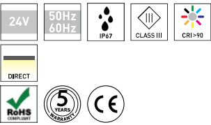
2005-102 NEON 10W IP67 TABELA DE PRODUTO E ESPECIFICAÇÕES TÉCNICAS - 2005-102 NEON Led Profissional 1010-SIDE 10W/m 24VDC IP67 CRI→90 5m/rolo 168LED/M
