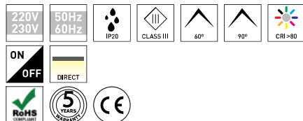
CAROLINE 10W - 100MM TABELA DE PRODUTO E ESPECIFICAÇÕES TÉCNICAS - CRI→80
