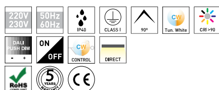
ORIS 50 LS SALIENTE OPAL TABELA DE PRODUTO E ESPECIFICAÇÕES TÉCNICAS - CRI>90
