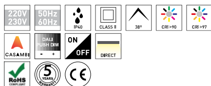
SPAR EFF. UNIVERSAL 24W TABELA DE PRODUTO E ESPECIFICAÇÕES TÉCNICAS - CRI>90
