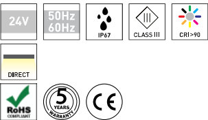
2005-102 NEON 10W IP67 TABLEAU DES PRODUITS ET SPÉCIFICATIONS TECHNIQUES - 2005-102 NEON LED Professionnel 1010-SIDE 10W/m 24VDC IP67 CRI→90 5m/rouleau 168LED/M
