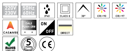
SPAR EFF. UNIVERSEL 28,4W TABLEAU DES PRODUITS ET SPÉCIFICATIONS TECHNIQUES - CRI→90
