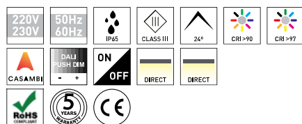
TYR 13W - IP65 TABLEAU DES PRODUITS ET SPÉCIFICATIONS TECHNIQUES - CRI->90
