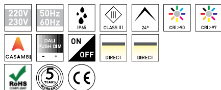
TYR 17W - IP65 TABLEAU DES PRODUITS ET SPÉCIFICATIONS TECHNIQUES - CRI->90
