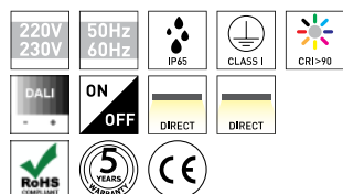
IRIS V ESTANCA 360° IP65 TABLA DE PRODUCTOS Y ESPECIFICACIONES TÉCNICAS - CRI→90
