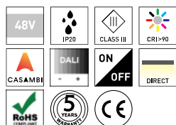
LAZULI 48V EVO TABLA DE PRODUCTOS Y ESPECIFICACIONES TÉCNICAS - CRI→90
